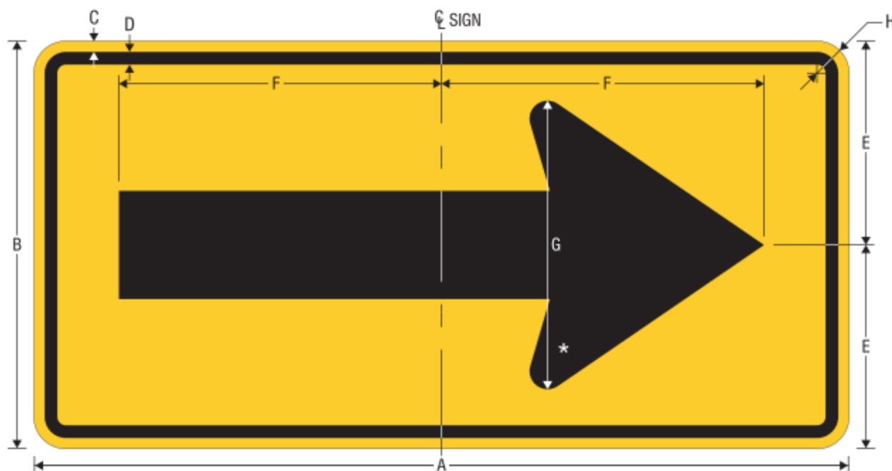
W1-6R
