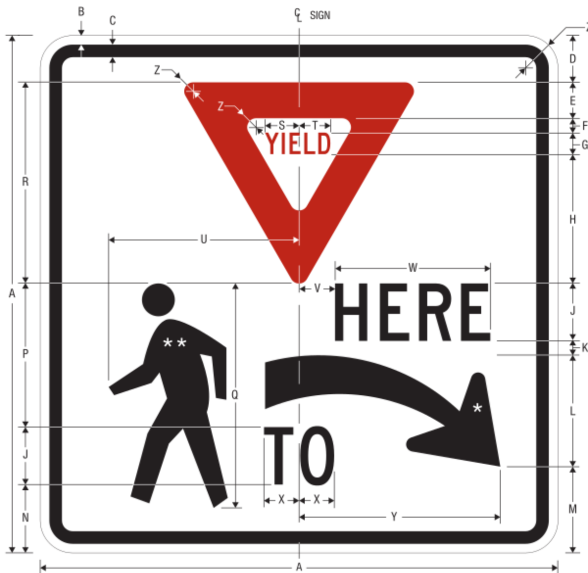
R1-5R
